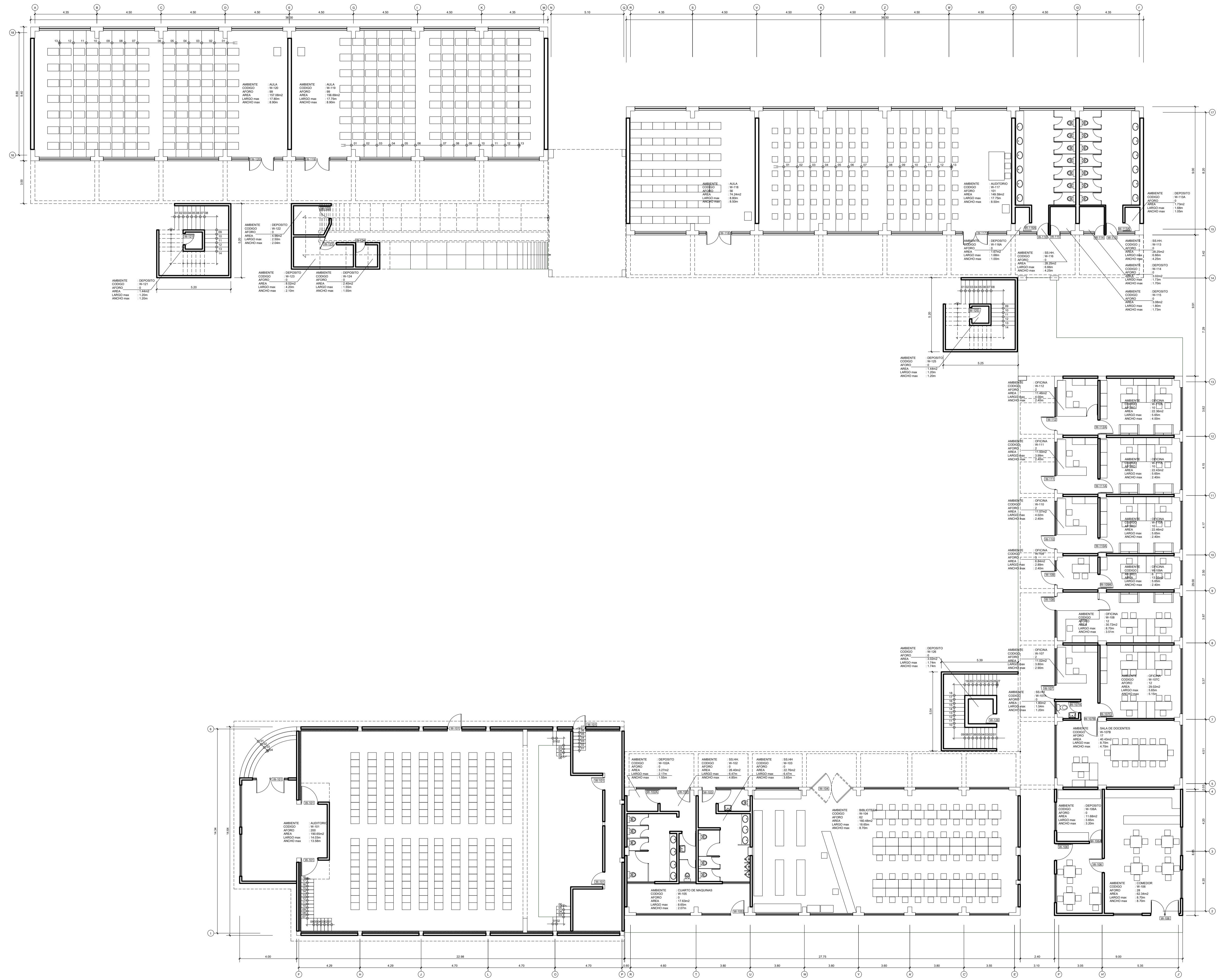
PRIMERA PLANTA AREA TECHADA = 2179.20m 2 AFORO = 733 ESCALA 1:100
